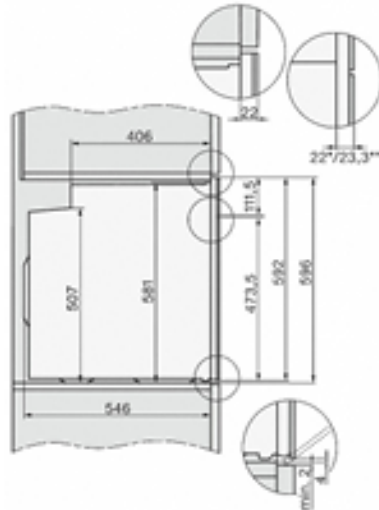
H2760B/BP, H28x0B/BP, H7x6xB/BP/BPX, installation drawings, GB, AUS
