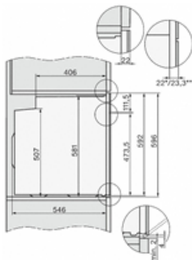
H2760B/BP, H28x0B/BP, H7x6xB/BP/BPX, installation drawings, GB, AUS
