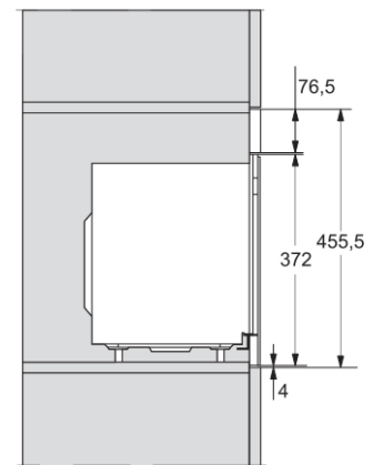
Seitenansicht M223xSC, AB45-2, Skizze
