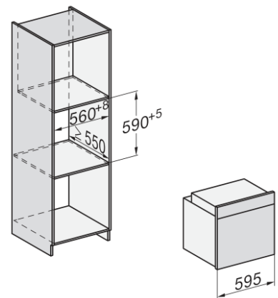
Einbau H7000 XL, Skizze
