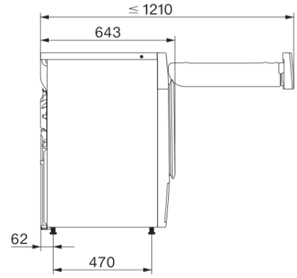
T1 Skizze, 5 Grad Blende, mit Sichtfenster, Maße in mm
