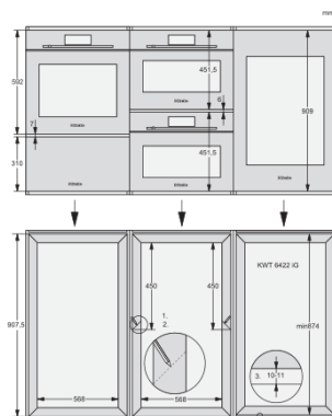
ENB1060, combination 60er & 32er ESW + 2x45er + KWT6422iG, Installation draw
