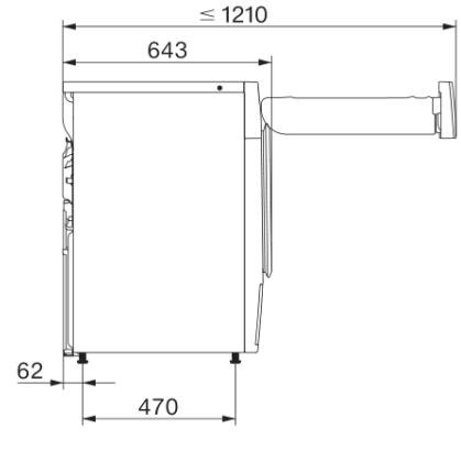
T1 Skizze, 5 Grad Blende, mit Sichtfenster, Maße in mm
